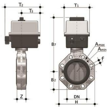
Дисковый затвор FK ПВХ с эл.приводом 24V AC/DC, EPDM, FIP d10" (DN250)
