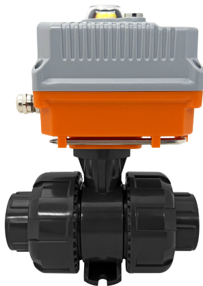
Шаровой кран IVKD PBX с эл.приводом 220V AC, муфтовые окончания, FKM, IPS d50 (DN40)
