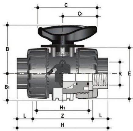
Шаровой кран для регулирования потока VKRFM с резьбовыми окончаниями (уплотнение EPDM) PP-H R1" (DN25)
