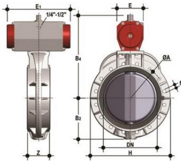
Дисковый затвор промышленного применения FK ПВХ с пневмоприводом НЗ, EPDM, FIP d355 (DN350)
