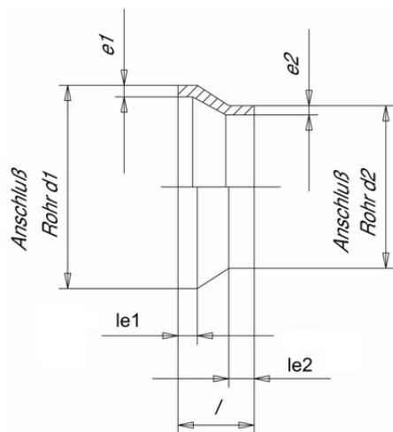
Муфта редукционная ПВДФ (Simona) 110x63 SDR33 PN10
