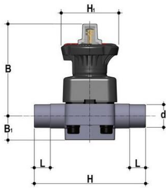
Мембранный клапан DK/L с втулочными окончаниями (уплотнение FKM / мембрана FKM) PP-H d32 (DN25)
