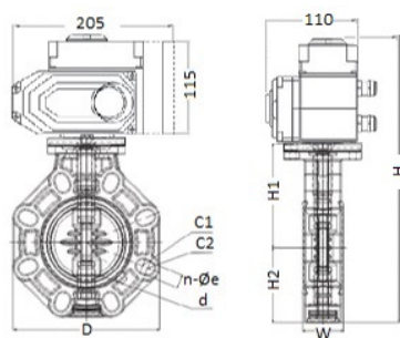
Дисковый затвор IFK ХПВХ с электрическим приводом 24V DC, FKM, IPS d140 (DN125)
