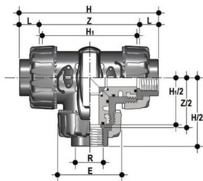
3-х ходовой шаровой кран ТКД ХПВХ с резьбовыми окончаниями, L-шар R2" (DN50)
