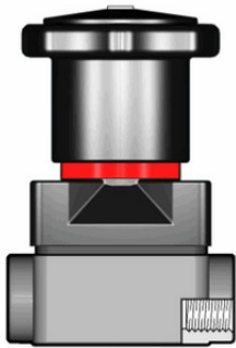
Компактный мембранный клапан ПВХ с пневмоприводом, СМ, EPDM, FIP R3/8" (DN12)
