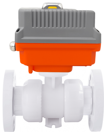
Шаровой кран IVKD ПВДФ с эл.приводом 24V DC, фланцевые окончания, FKM, IPS d110 (DN100)
