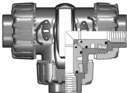
3-х ходовой шаровой кран ТКД ХПВХ с резьбовыми окончаниями, Т-шар R1/2" (DN15)
