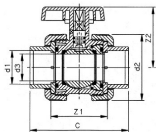
Шаровой кран ПВХ промышленного применения с муфтовыми окончаниями, EPDM, VDL d90 (DN80)
