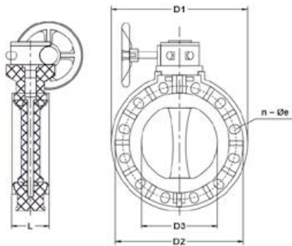
Затвор дисковый промышленный с редуктором ХПВХ IPS (Model B) d16"(DN400)
