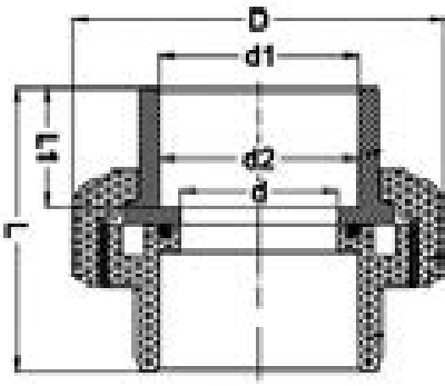
Муфта ХПВХ IPS d32 PN16
