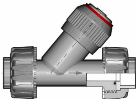
Угловой обратный клапан VRUIV PBX с разборными муфтовыми окончаниями, FKM, FIP d20 (DN15)
