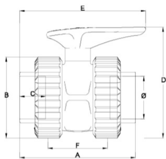
Шаровой кран ПВХ промышленного применения с муфтовыми окончаниями, EPDM, Hidroten d63 (DN50)
