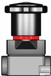
Компактный мембранный клапан CM ПВХ с пневмоприводом ДвД, резьбовые окончания, EPDM, FIP R1/2" (DN15)
