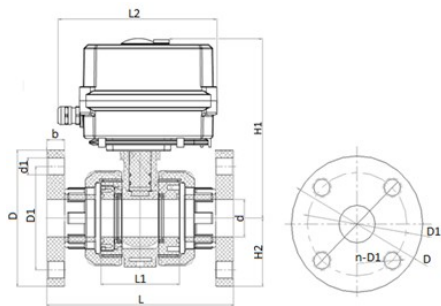
Шаровой кран IVKD ХПВХ с эл.приводом 24V DC, фланцевые окончания d32 (DN25)
