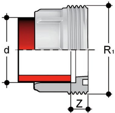
Муфтовая вставка ПВДФ d32 SDR21 PN16
