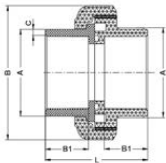
Муфта разборная для стыковой сварки PP-H IPS d32 PN 10
