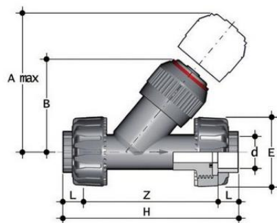
Угловой обратный клапан VRUIV PBX с разборными муфтовыми окончаниями, FKM, FIP d16 (DN10)
