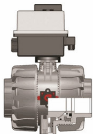
Шаровой кран VKD ПВХ с эл.приводом 90-240V, муфтовые окончания, DN65-100, FKM, FIP d110 (DN90)
