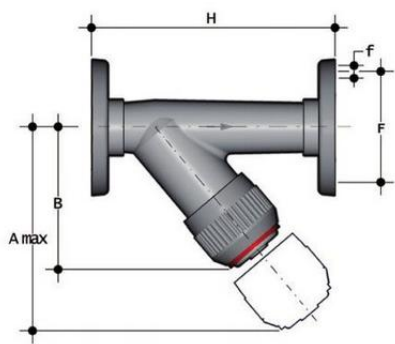
Грязевый фильтр RVOT PBX с фланцевыми окончаниями, EPDM, FIP d90 (DN80)
