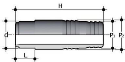
Шланговый адаптер PP-H FIP d20 PN10
