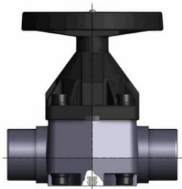
Мембранный клапан VM ПВДФ с втулочными окончаниями d110 (DN90)
