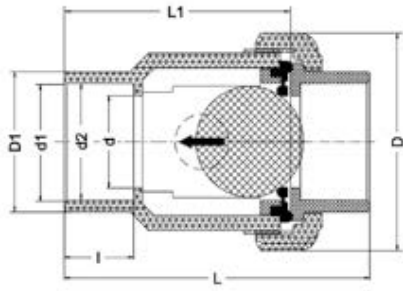
Обратный клапан шаровой с одним разборным соединением, муфтовые окончания PP-H IPS (FKM) d50 (DN40)
