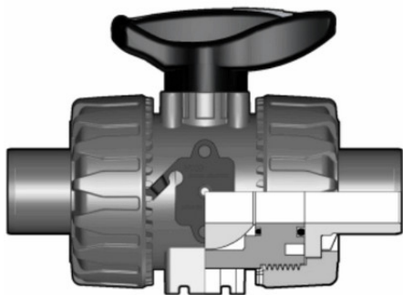
Шаровой кран промышленного применения VKD со втулочными окончаниями (уплотнение FKM) PP-H d20 (DN15)
