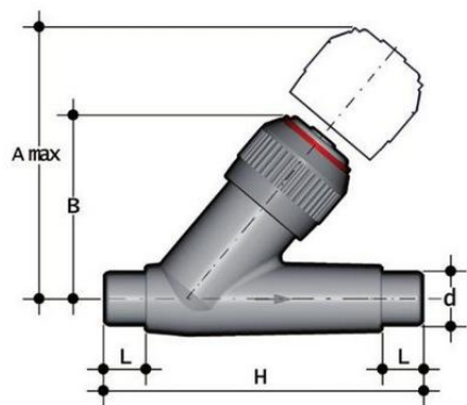
Угловой обратный клапан VRDV PBX с втулочными окончаниями, EPDM, FIP d50 (DN40)
