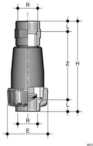
Донный клапан VZFV ПБХ с резьбовыми окончаниями, EPDM, FIP R1" (DN25)
