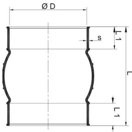
Шаровая манжета с лентой PPs d250
