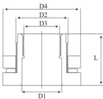
Соединитель с цистерной, ILIFV ПВХ IPS d32
