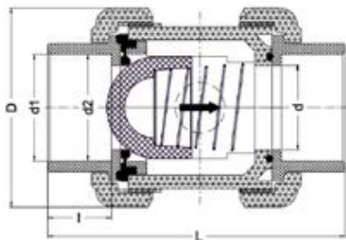
Пружинный обратный клапан ISSE ПBX; с муфтовыми окончаниям, EPDM, IPS d75 (DN65)
