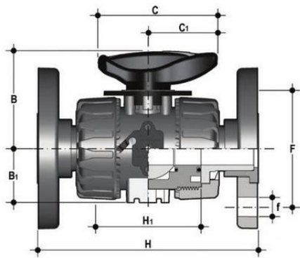
Шаровой кран для регулирования потока VKR ПВДФ с фланцевыми окончаниями d50 (DN40)
