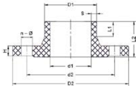
Фланцевое соединение жесткое для стыковой сварки PP-H IPS d140 PN10
