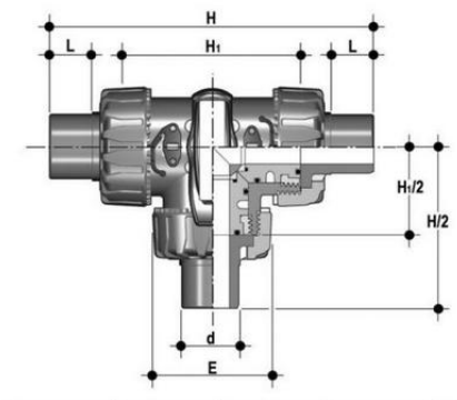
3-х ходовой шаровой кран ТКД с втулочными окончаниями L-шар (уплотнение FKM) PP-H d32 (DN25)
