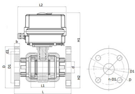
Шаровой кран IVKD ПВДФ с эл.приводом 24V DC, фланцевые окончания, EPDM, IPS d110 (DN100)
