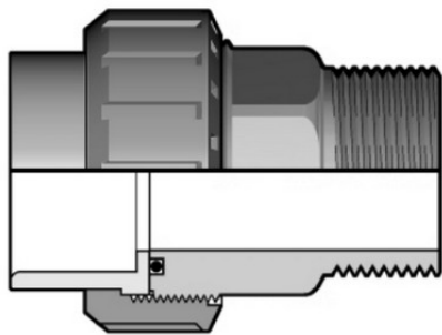
Муфта разборная с НР ПВХ FIP 63x2
