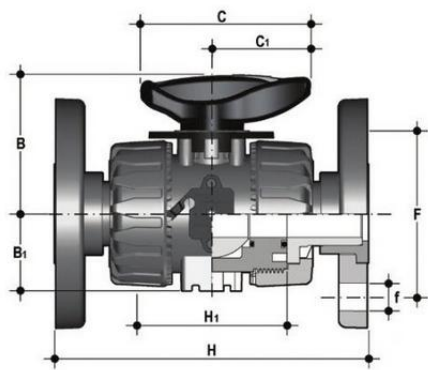
Шаровой кран ПВХ для регулирования потока VKR с фланцевыми окончаниями, EPDM, FIP d32 (DN25)
