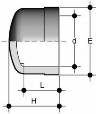
Заглушка клеевая ПВХ FIP d20
