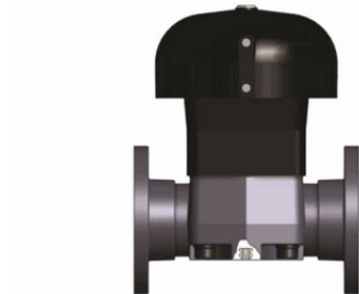
Мембранный клапан VM с пневмоприводом НО, PN10 с фланцевыми окончаниями (уплотнение EPDM/мембрана EPDM) PP-H d110 (DN100)
