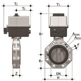
Дисковый затвор FK с эл.приводом 24V AC/DC (уплотнение FKM) PP-H d140 (DN125)
