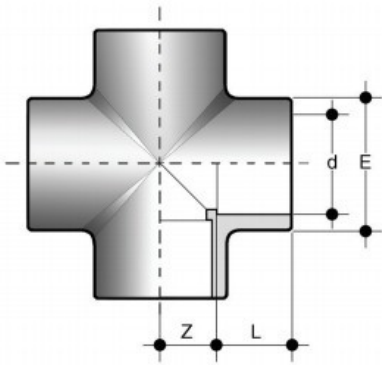
Крестовина клеевая ПВХ FIP d63
