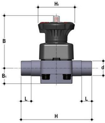
Мембранный клапан DKDV ПВХ с втулочными окончаниями, FKM, FIP d40 (DN32)
