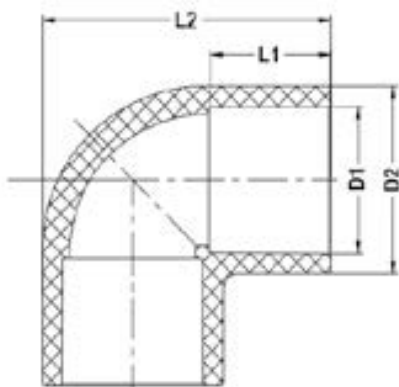
Отвод 90° ХПВХ IPS (Model A) d110 PN16
