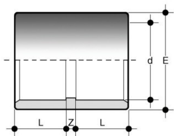
Муфта соединительная ПВХ FIP d110
