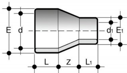
Муфта редукционная ПВХ FIP 250x140
