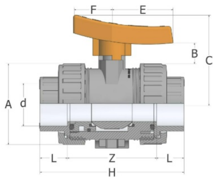
Кран шаровый ХПВХ муфтовый промышленный EPDM Comer d63 (DN50)
