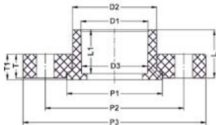
Фланец свободный с буртом ХПВХ IPS (Model A) - комплект d20 PN16
