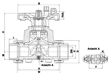
Мембранный клапан PBX с муфтовыми окончаниями, FKM, Praher Plastics d32 (DN25)
