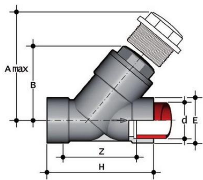
Угловой обратный клапан VR с муфтовыми окончаниями, (уплотнение EPDM) PP-H d90 (DN80)
